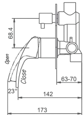
DMWD1 - Demos Wall Mixer w\ Diverter - Chrome
